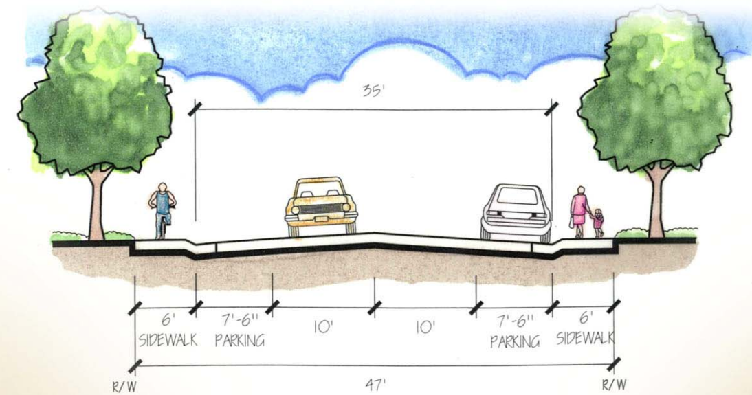
LOCAL STREET / CUL DE SAC
